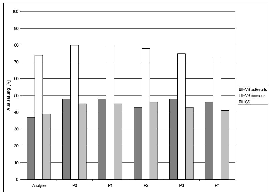
6: Vergleich der Auslastungen im Gesamtnetz
