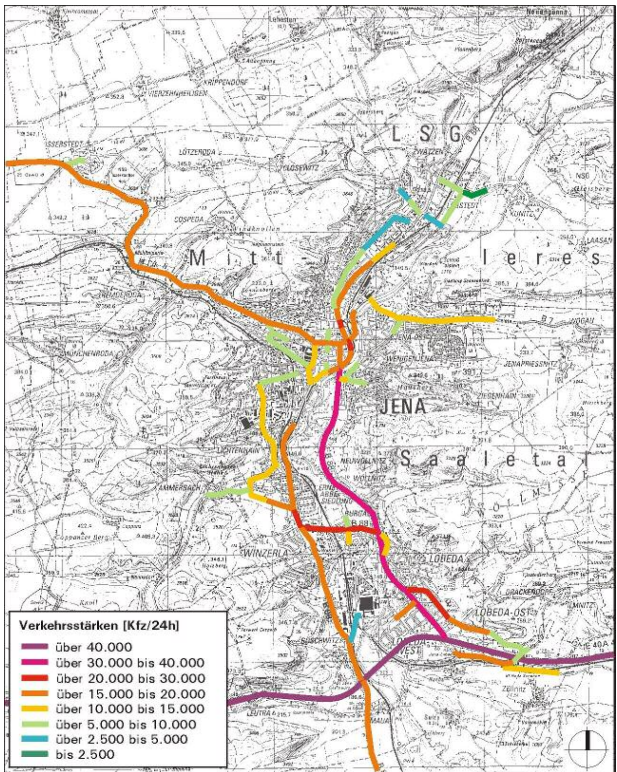
1: Verkehrsmengenkarte für das Hauptverkehrsstraßennetz [Kfz/24h] (Quelle: Knotenpunkt- und Querschnitterhebungen aus den Jahren 1998 und 2001)
